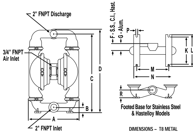
DIMENSIONS - T8 METAL
